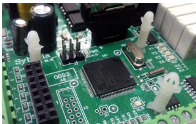
Рисунок 4. (Установка стоек)
